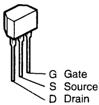
2SK161
