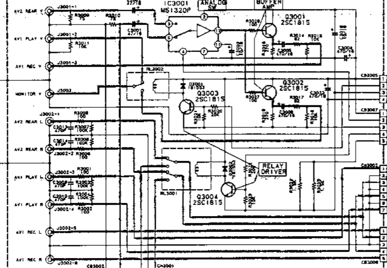
AV FRONT P. C. Board
