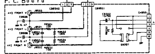
AV FRONT P. C. Board
