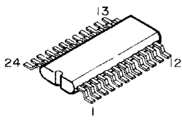
μPD449G: IC204
