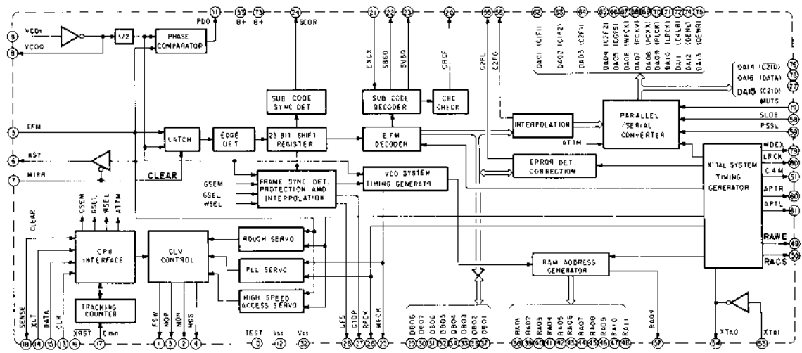
μPD449G: IC204
