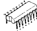
TD62504
