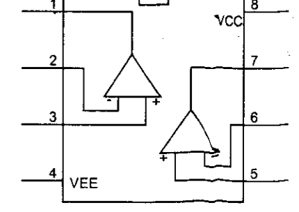
IC43: LT082
