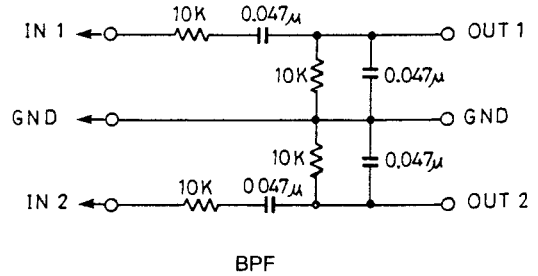
BPF
