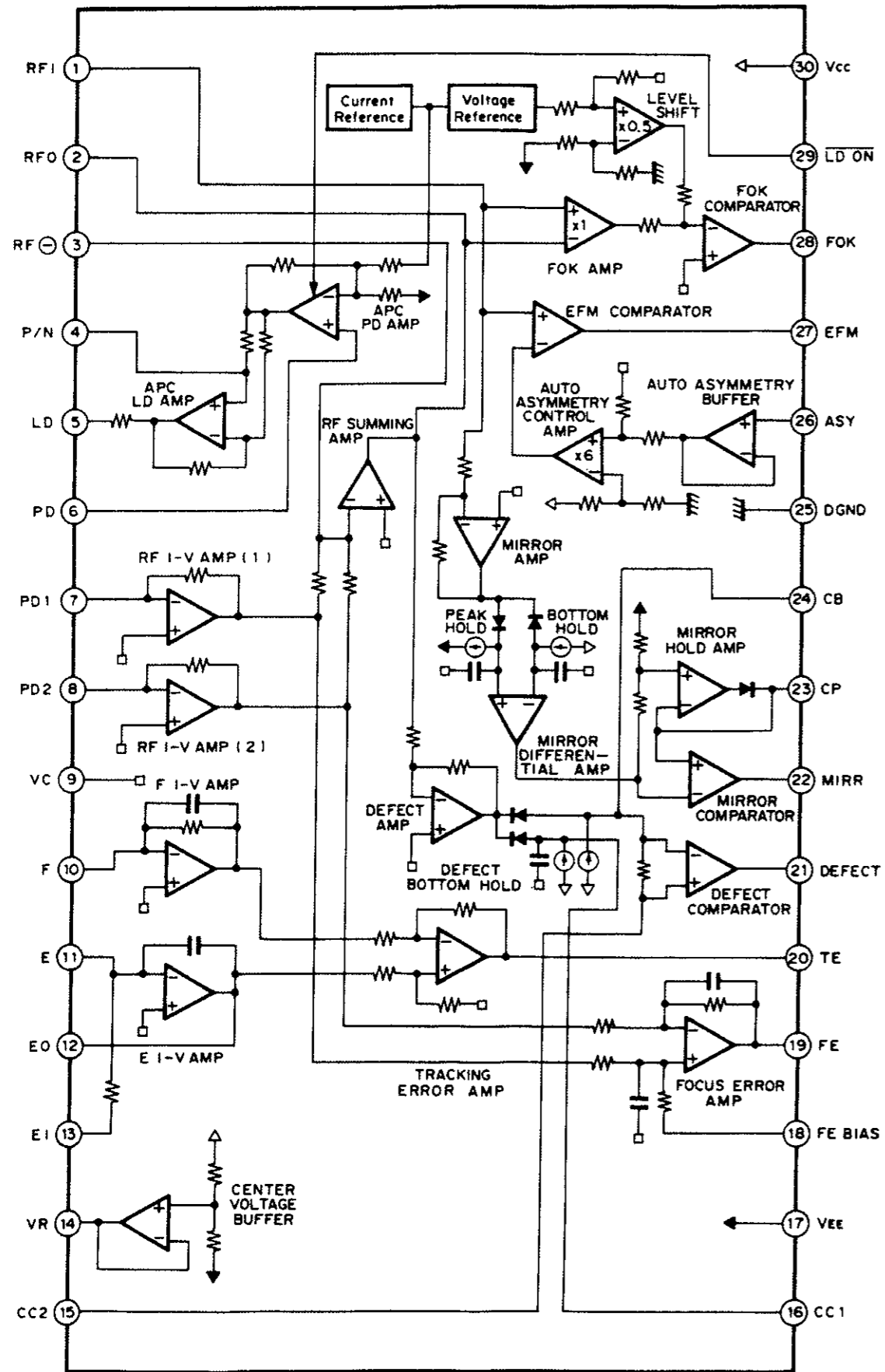
Q101: CXA1081M
