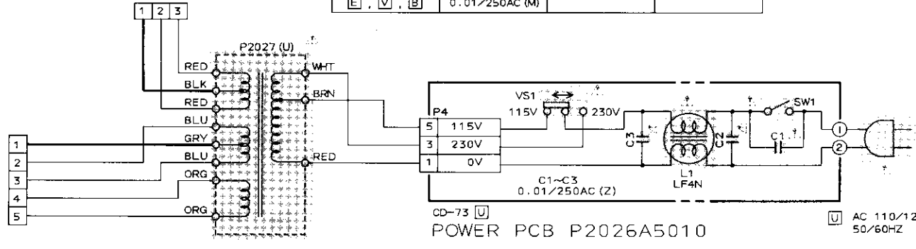
POWER PCB P2026A5010
