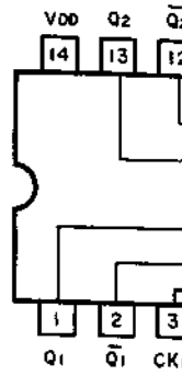
Fig. 13.10 D-Type Flip-Flop C-MOS IC \mu PD4013BC
