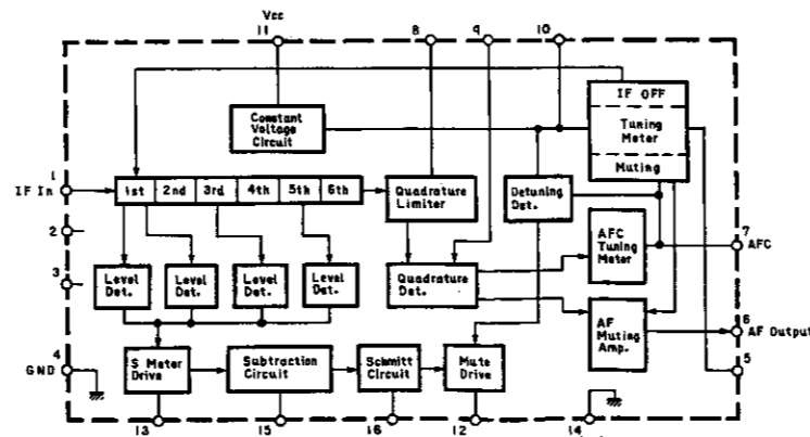
Fig. 7.1.9 FM IF Amp. & Detector IC LA1285
