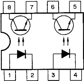
Fig. 8.1.3. Photo Coupler IC TLP621-2
