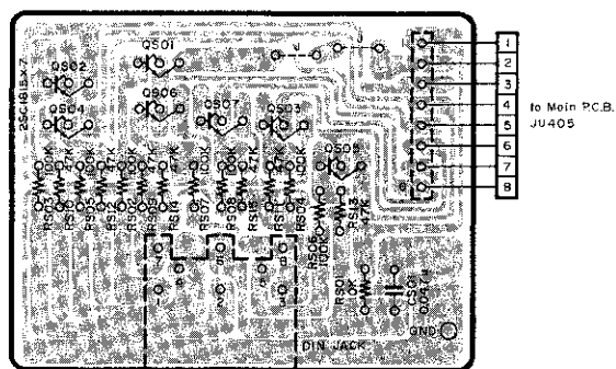
7.12. Voltage Selector P.C.B. Ass'y
