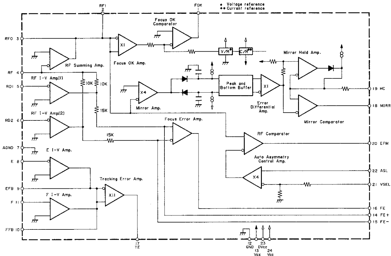
Fig. 8.1.13. RF Amp. IC CX20109
