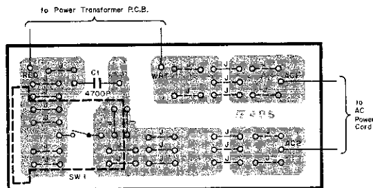
7.3. Power Switch P.C.B. Ass'y
