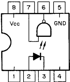
Fig. 8.1.4. Photo Coupler IC TLP552
