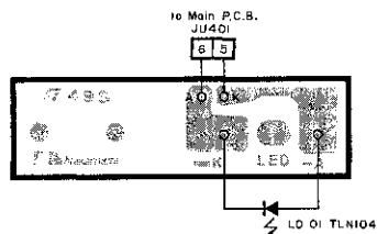
7.2. Photo Diode P.C.B. Ass'y
