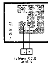
7.6. Inner End Switch P.C.B. Ass'y
