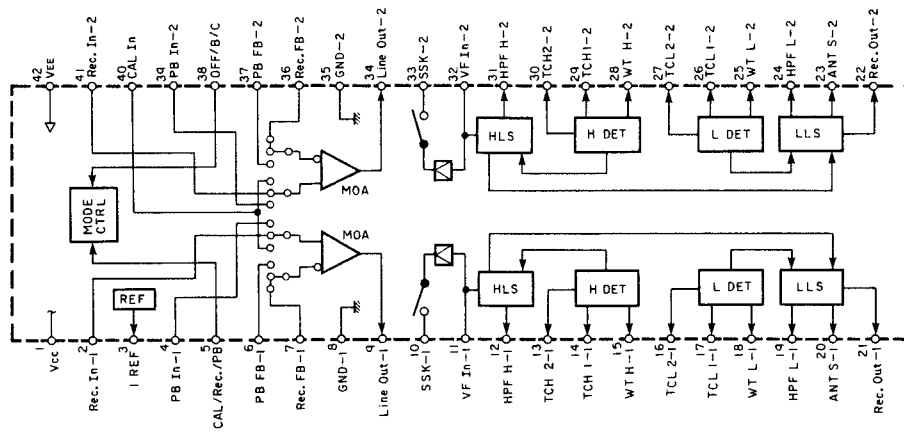
Fig. 9.1.3 Dolby NR IC CX20188
