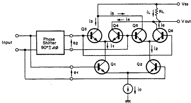
Fig. 2.1.26 Quadrature Detector Circuit
