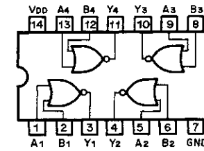
Fig. 10.7 NOR Gate C-MOS IC μPD4001C
