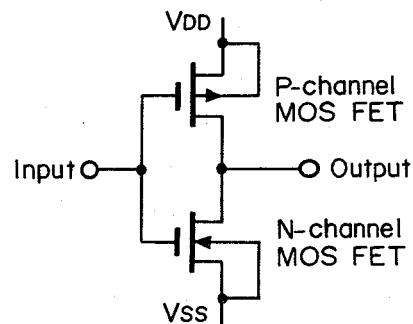
Fig. 2.1.1 C-MOS Inverter
