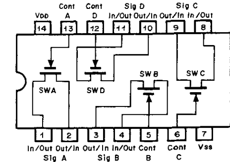
Fig. 10.10 Bilateral Switch C-MOS IC μPD4066C
