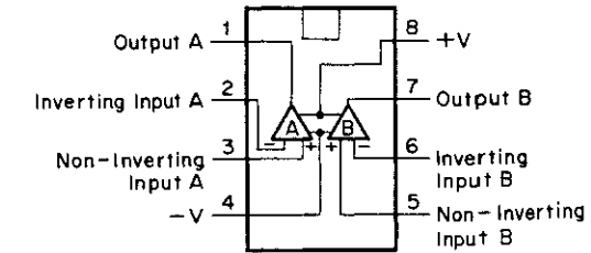
Fig. 10.8 OP Amp. IC RC4558 and RC4559
