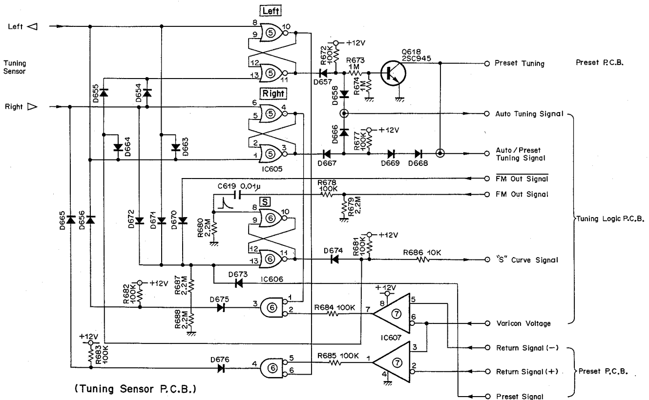
Fig. 2.4.11 Auto-Tuning Circuit
