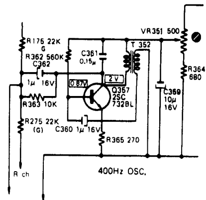
Fig. 2.21 400Hz Osc. Circuit Diagram
