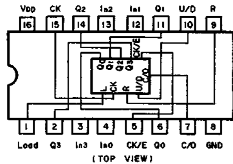
Fig. 13.14 BCD Up/Down Counter C-MOS IC TC4510BP
