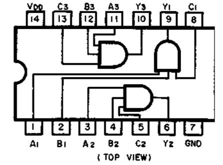
Fig. 13.12 AND Gate C-MOS IC \mu PD4073
