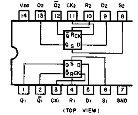
Fig. 13.13 D-Type Flip-Flop C-MOS IC
