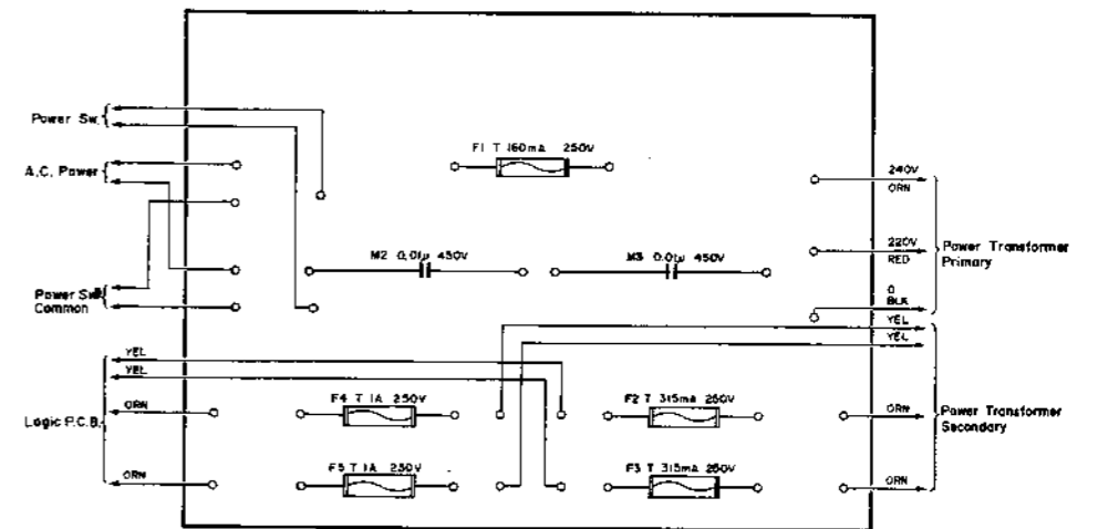
Fig. 7.6.4 220 V Class 2
