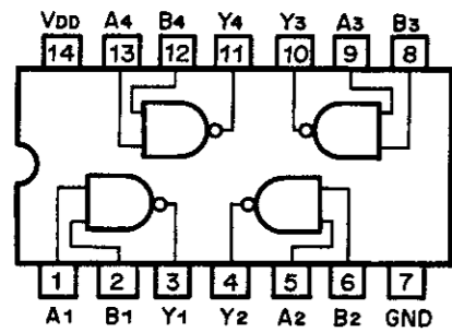
Fig. 13.5 C-MOS IC \mu PD4011C
