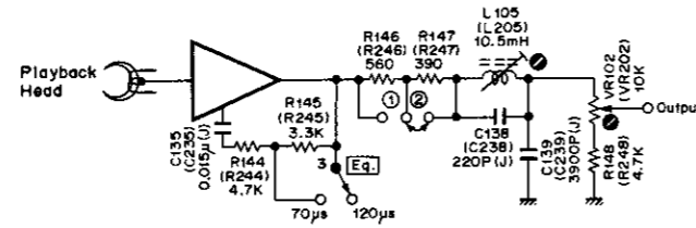
Fig. 6.1.13 Playback Amp.
