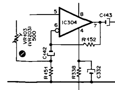
Fig. 6.2.6 4. Meter Level (15 kHz)
