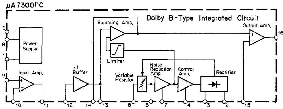
Fig. 13.3 Dolby NR IC \mu A7300PC
