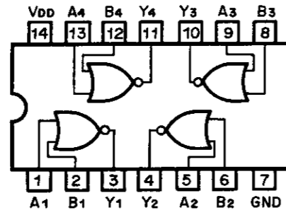
Fig. 13.6 C-MOS IC \mu PD4001C
