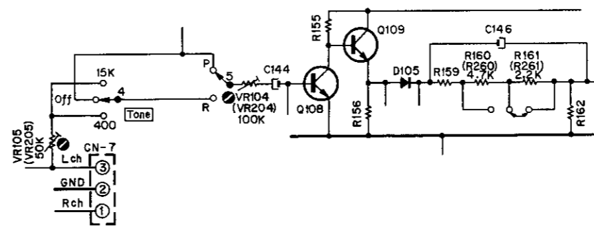
Fig. 6.1.5 3. Meter Level
