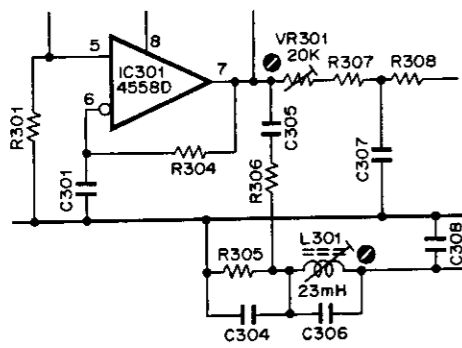
Fig. 6.1.3 2. Tone Calibration
