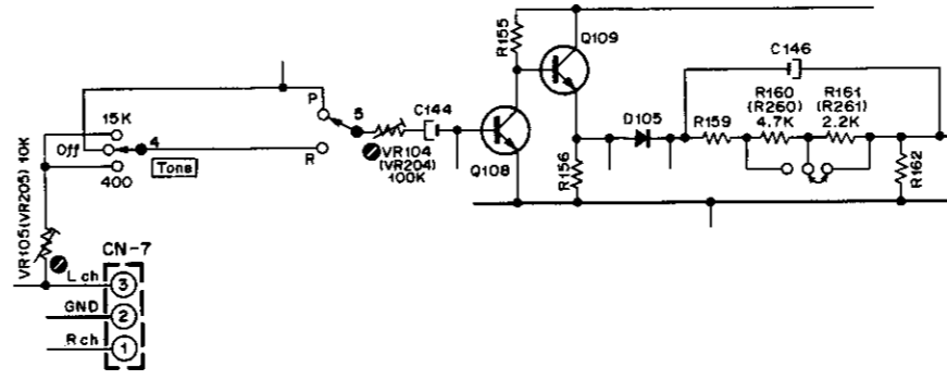
Fig. 6.2.5 3. Meter Level (400 Hz)
