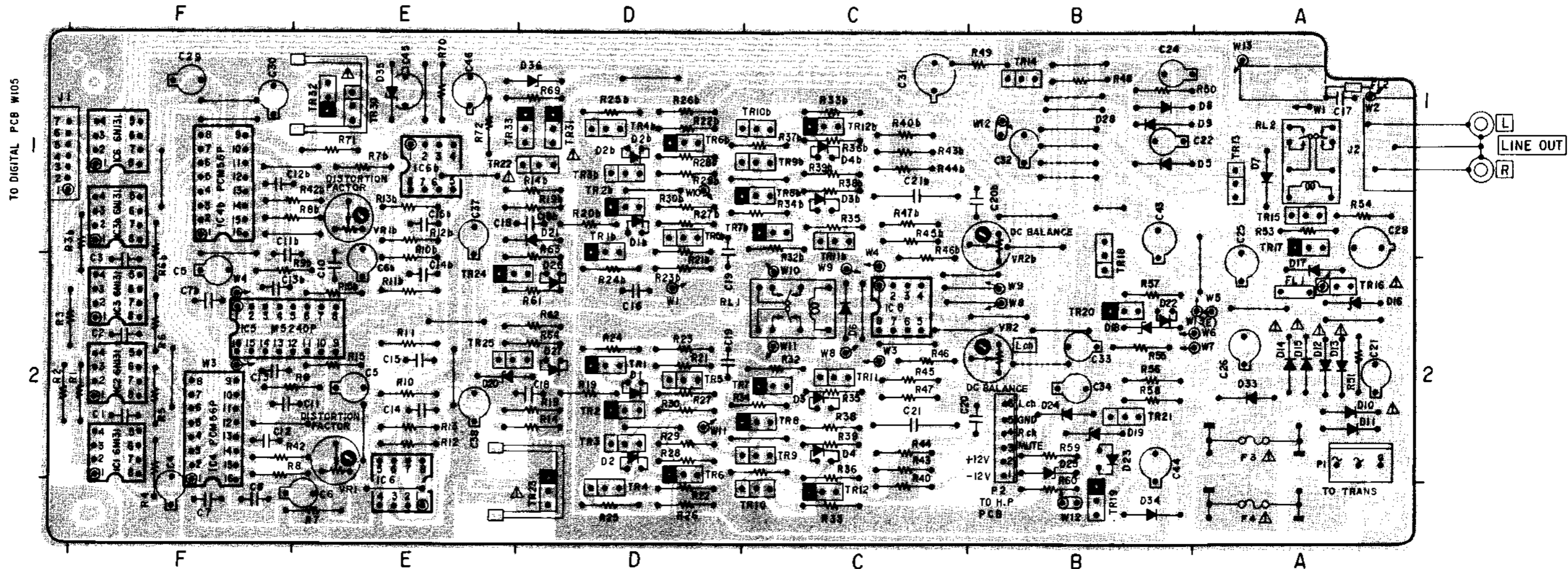
ANALOG PCB P2026B5040 (JI)
