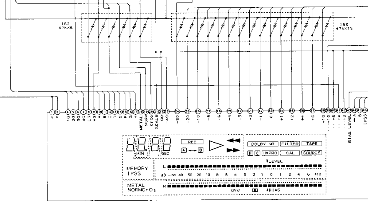
オペレーション基板 OPERATION PCB T2107A502B
