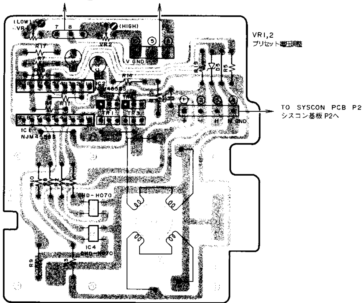
MOTOR PCB モーター基板 M3103C726A (J2)
