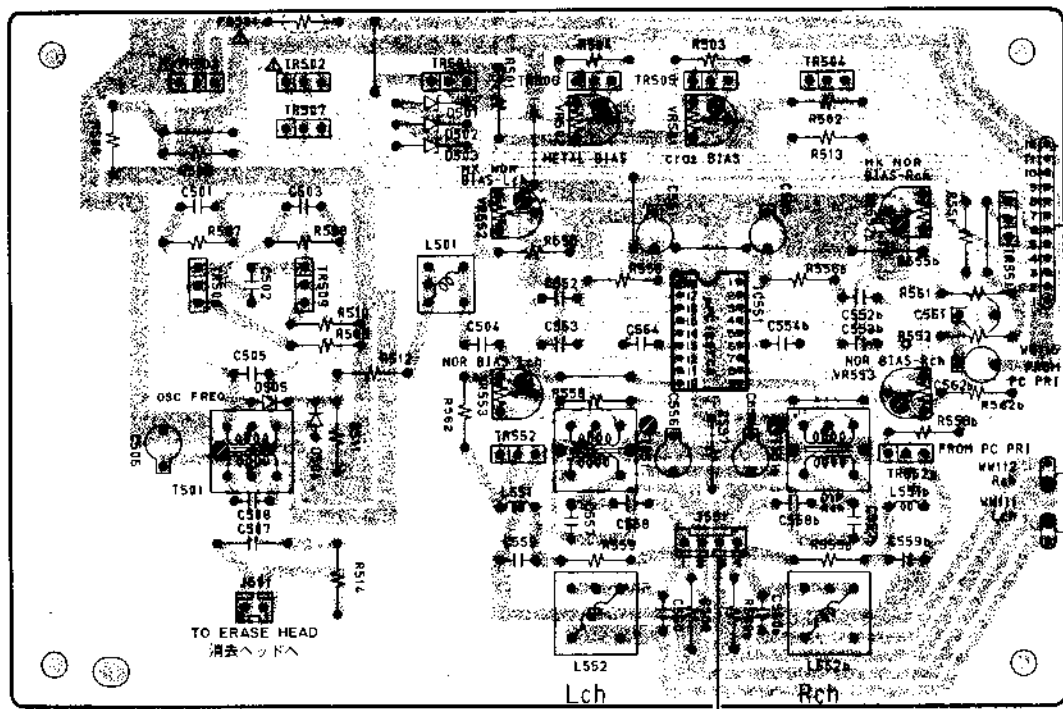
OSC PCB オシレータ基板 T2107A501B
