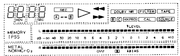
オペレーション基板 OPERATION PCB T2107A502B
