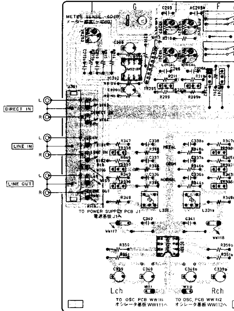
PREAMP PCB T2107A501A プリアンプ基板
