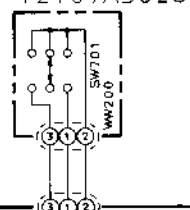
リールセンサー (R) 基板 REEL SENSOR (R) PCB T2069D5020 リールセンサー (L) 基板 REEL SENSOR (L) PCB T2069D5010 タイマー基板 TIMER PCB T2107A502C
