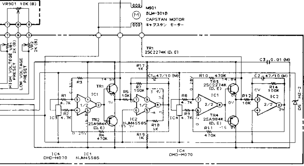
モーター基板 MOTOR PCB M3103C726A
