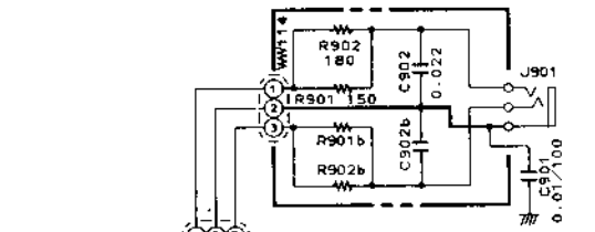
ヘッドホン基板 HEAD PHONE PCB T2107A501C T2107028
