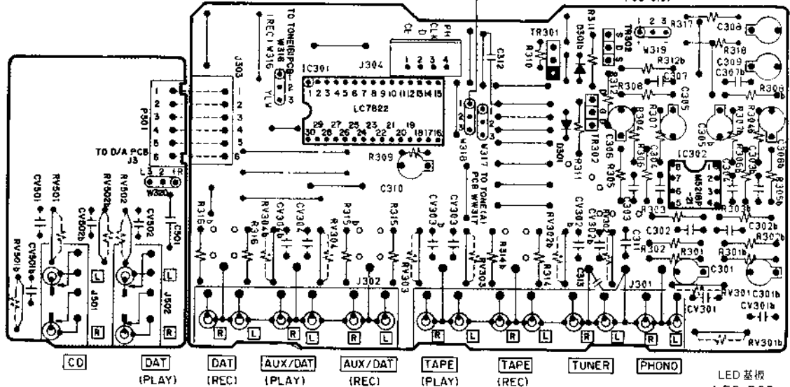
ジャック基板 JACK PCB A2054A502F
