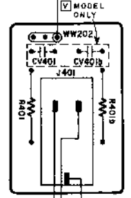
PHONE PCB A2054A501E ヘッドホーン基板
