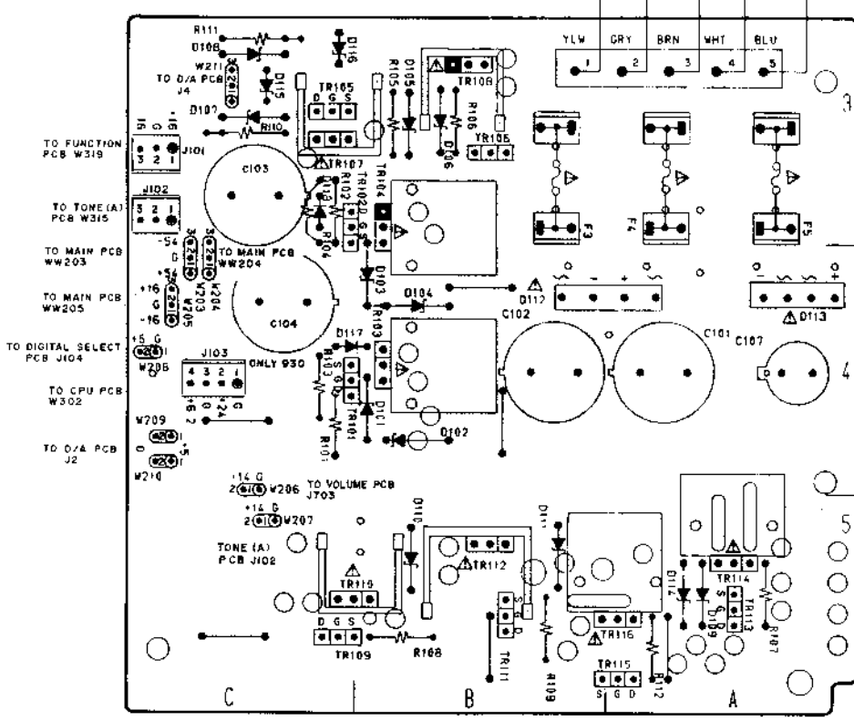
POWER SUPPLY PCB A2054A501B 電源基板
