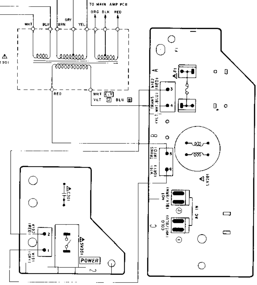
POWER SW PCB A2054A501D 電源スイッチ基板
