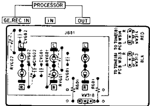
プロセッサー基板 PROCESSOR PCB A2054A502G
