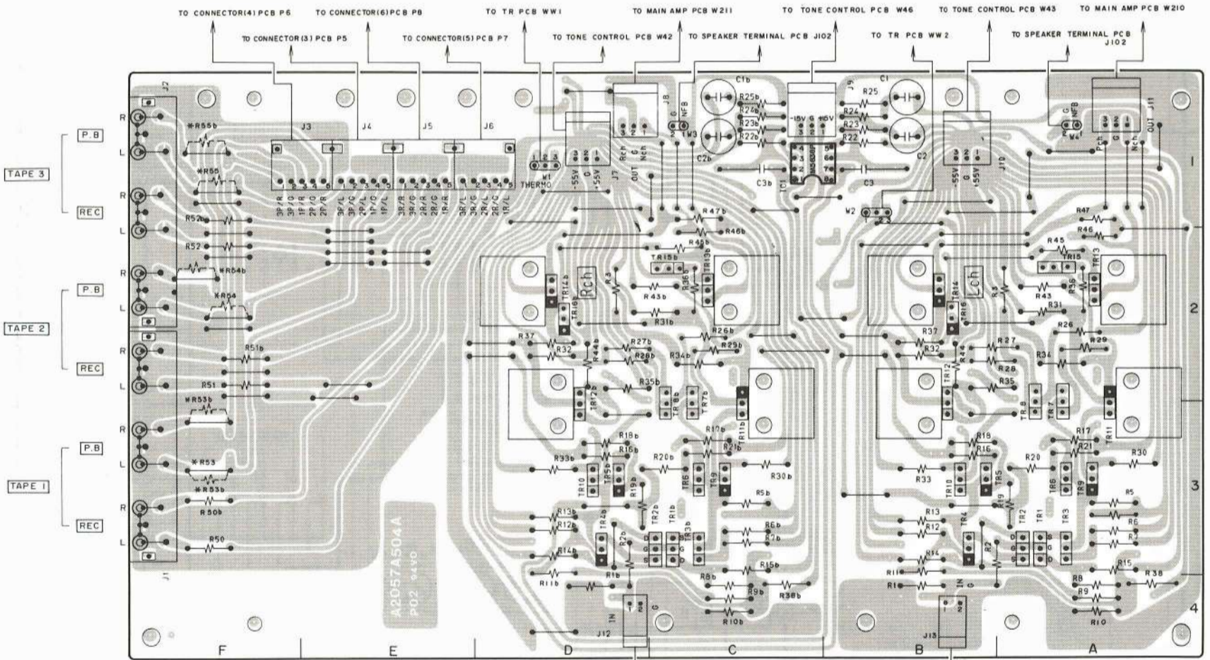
V-AMP PCB A2057A504A
