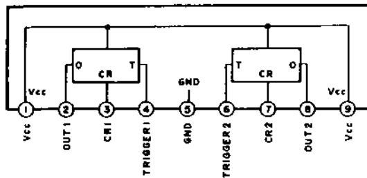
BA235A (DUAL MONO MULTI)
