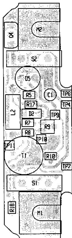
Gedruckte Schaltung EK 2014 TV, DC/DC-Wandler, Bestückungsseite Printed circuit board EK 2014 TV, DC/DC converter, equipped side
