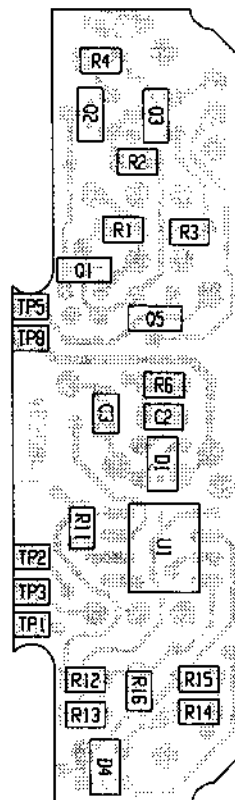
Gedruckte Schaltung EK 2014 TV, DC/DC-Wandler, Lötseite Printed circuit board EK 2014 TV, DC/DC converter, solder side
