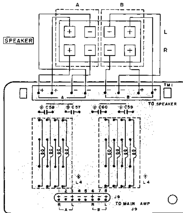
SPEAKER P.C.B
