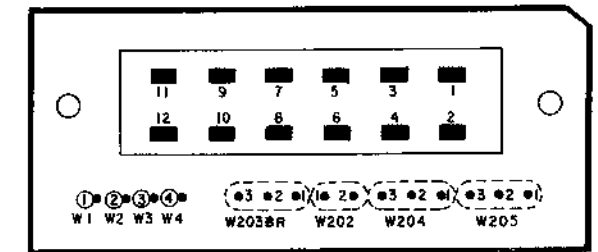
PLUG PCB PCB-015-4 プラグ基板
