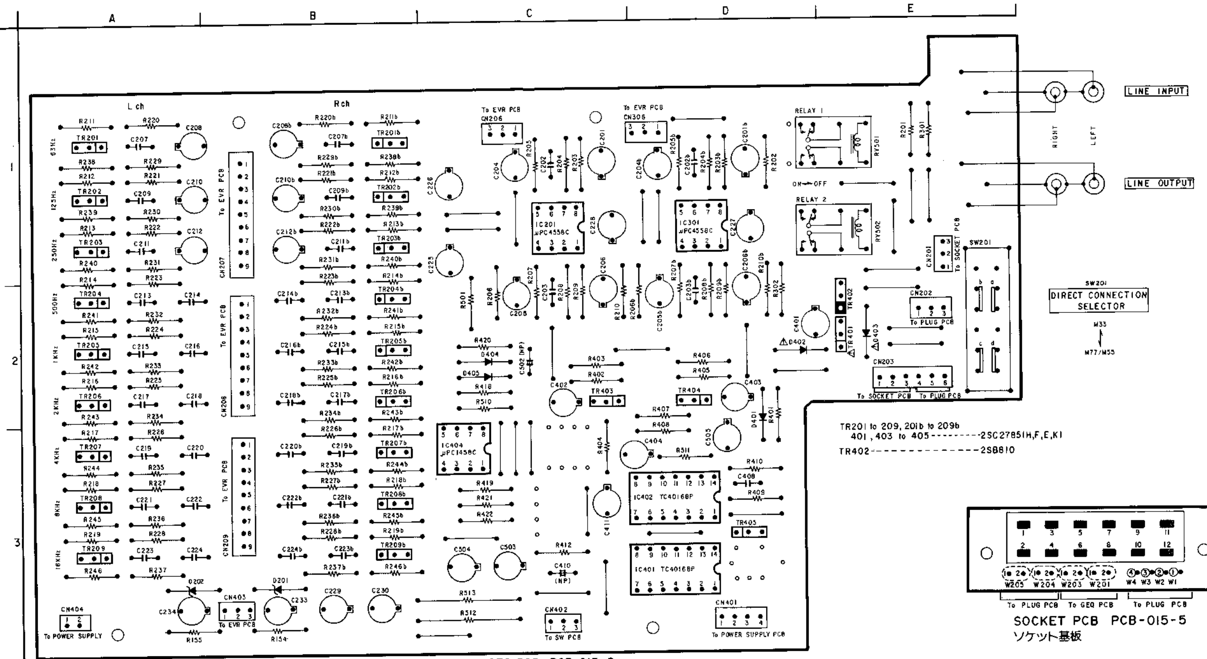
GEQ PCB PCB-015-2 GEQ基板
