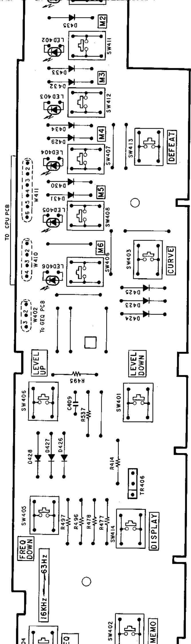
SW PCB PCB-016-3 スイッチ基板
