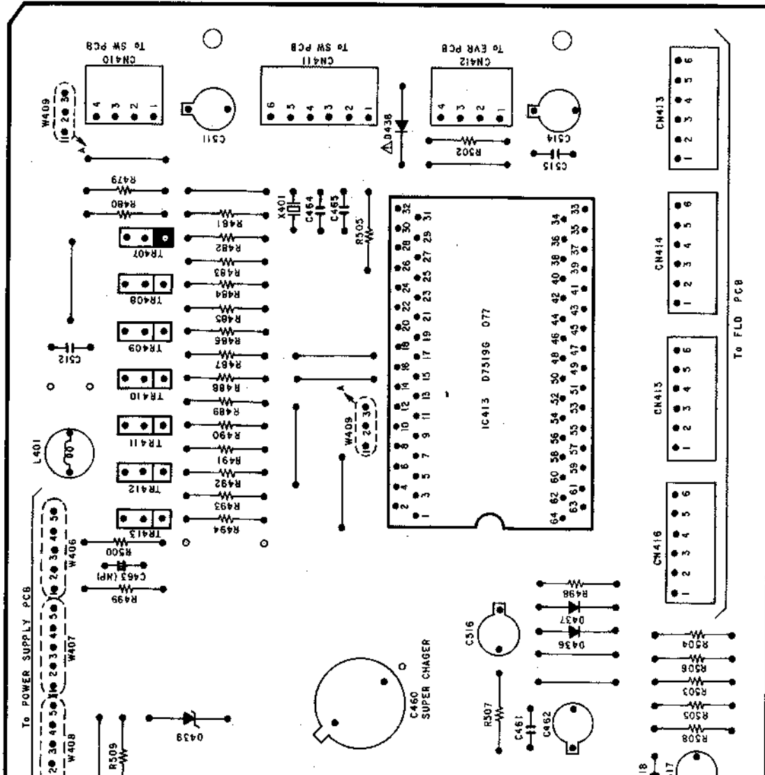
CPU PCB PCB-015-3 CPU基板
