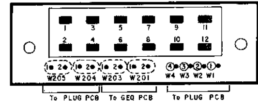
SOCKET PCB PCB-015-5 ソケット基板
