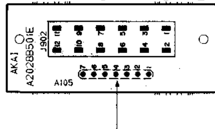
ソケット基板 SOCKET PCB A2028B501E
