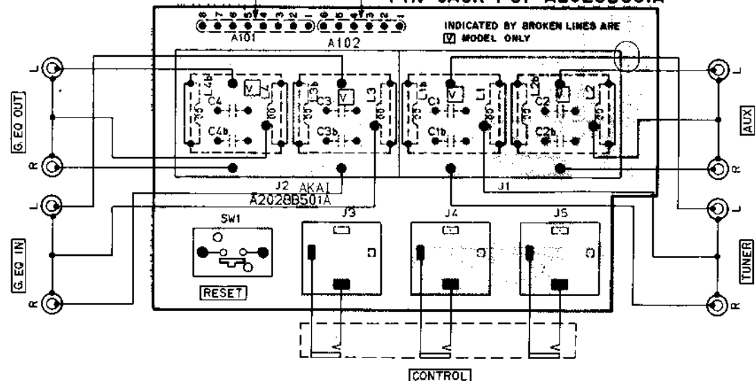
ピンジャック基板 PIN JACK PCB A2028B501A
