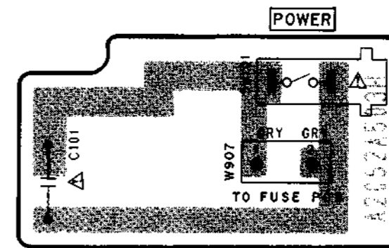
POWER SW PCB A2052A503H
