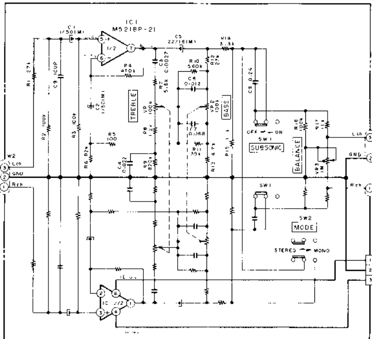
PRE AMP PCB A2052A502A
