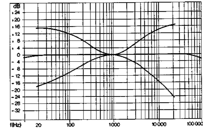
Fig. 9 Wirkungsweise der physiologischen Lautstärkeregelung. 0 dB = Lautstärkereglern offen
