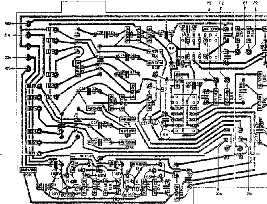
Regelverstärkerplatte
