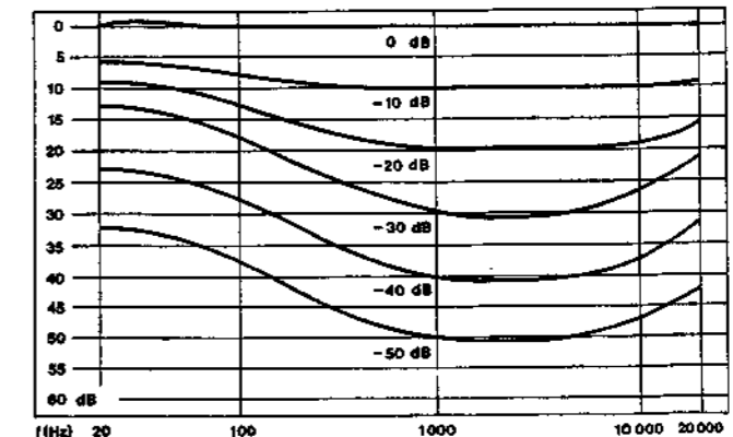
Fig. 9 Wirkungsweise der physiologischen Lautstärkeregelung. 0 dB = Lautstärkereglern offen
