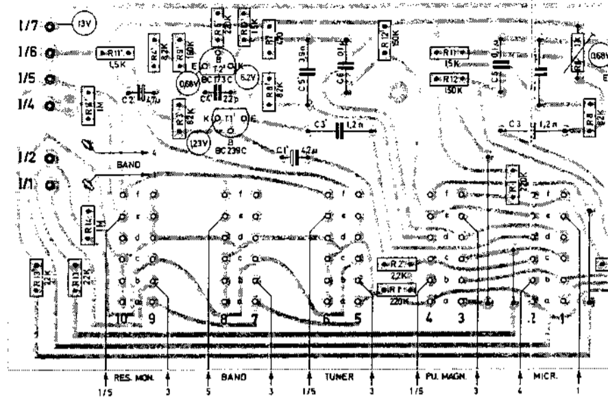
Vorverstärkerplatte
