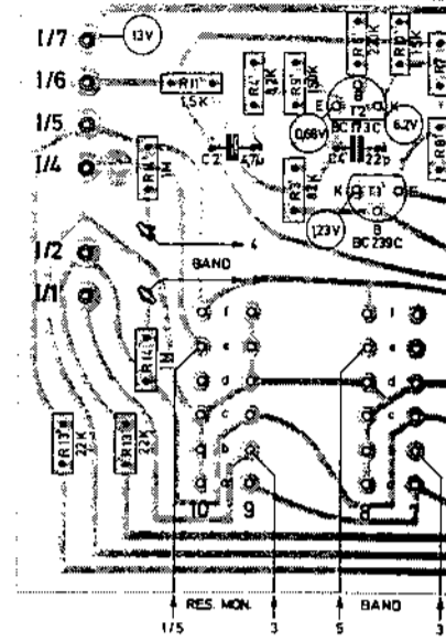
Vorverstärkerplatte
