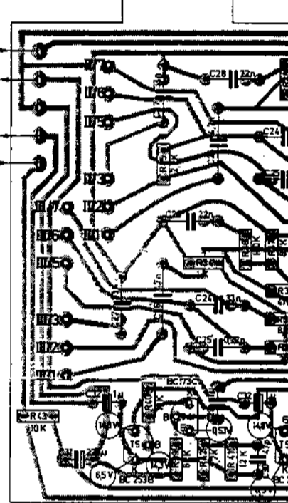
Regelverstärkerplatte
