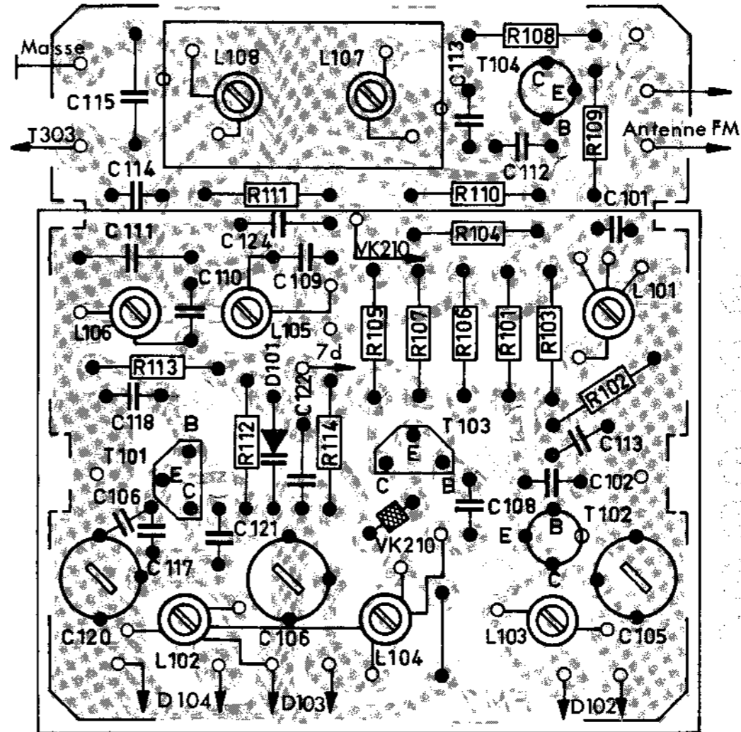
Fig. 8 Dioden-Platte (Bestückungsseite)
