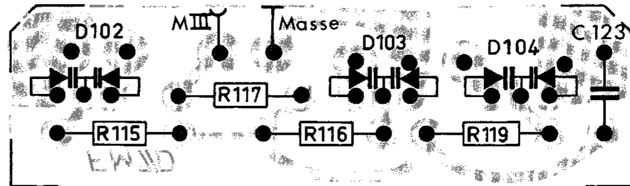
Fig. 8 Dioden-Platte (Bestückungsseite)
