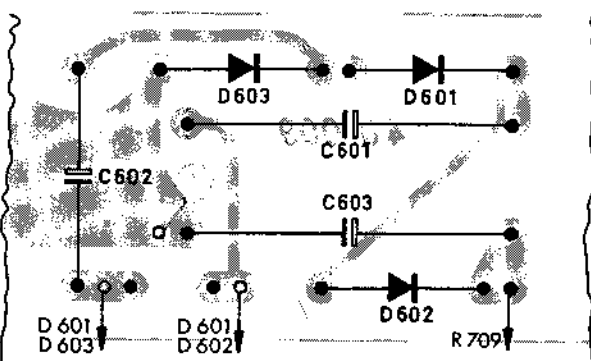
Fig. 2 Spannungswandler-Platte (Bestückungsseite)
