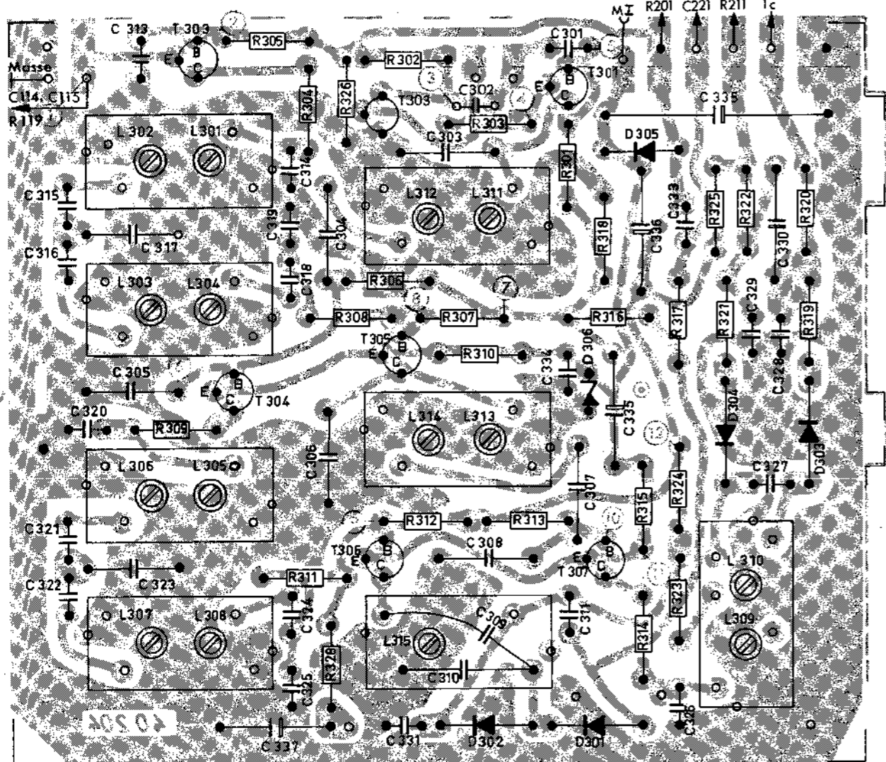
Fig. 3 ZF-Platte (Bestückungsseite)
