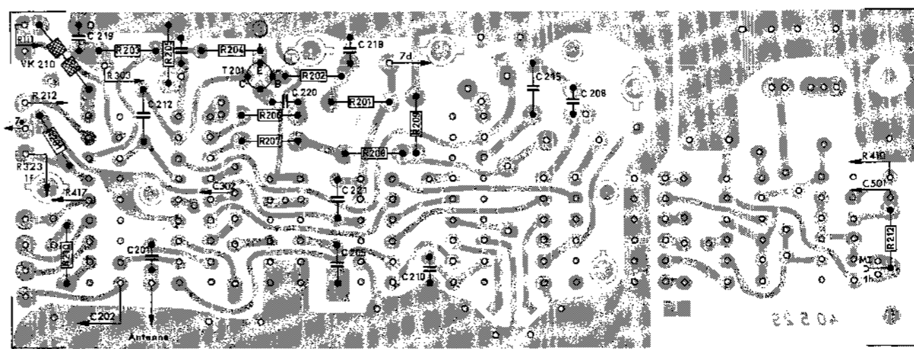
Fig. 5 Tastenschalter-Platte (Bestückungsseite)
