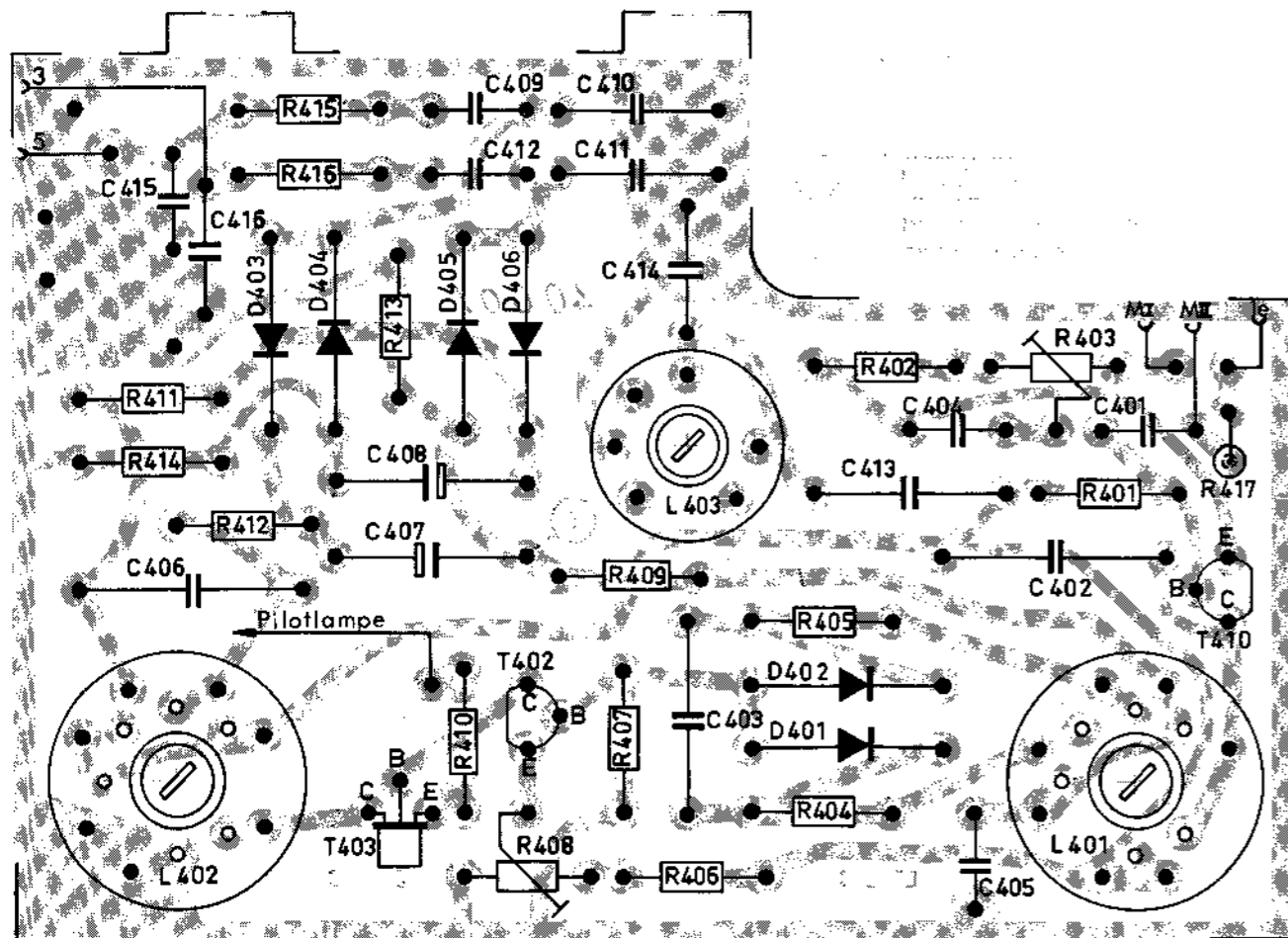
Fig. 6 Decoder-Platte (Bestückungsseite)
