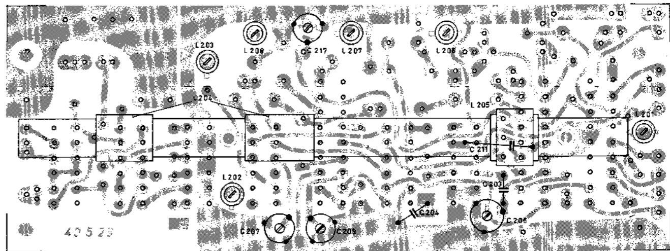
Fig. 4 Tastenschalter-Platte (Leiterseite)
