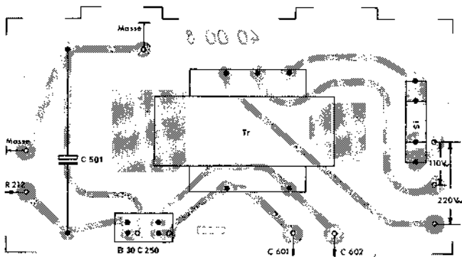
Fig. 1 Netzteil-Platte (Bestückungsseite)
