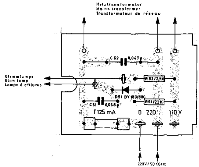
Fig. 3 Netzplatte (Bestückungsseite)
