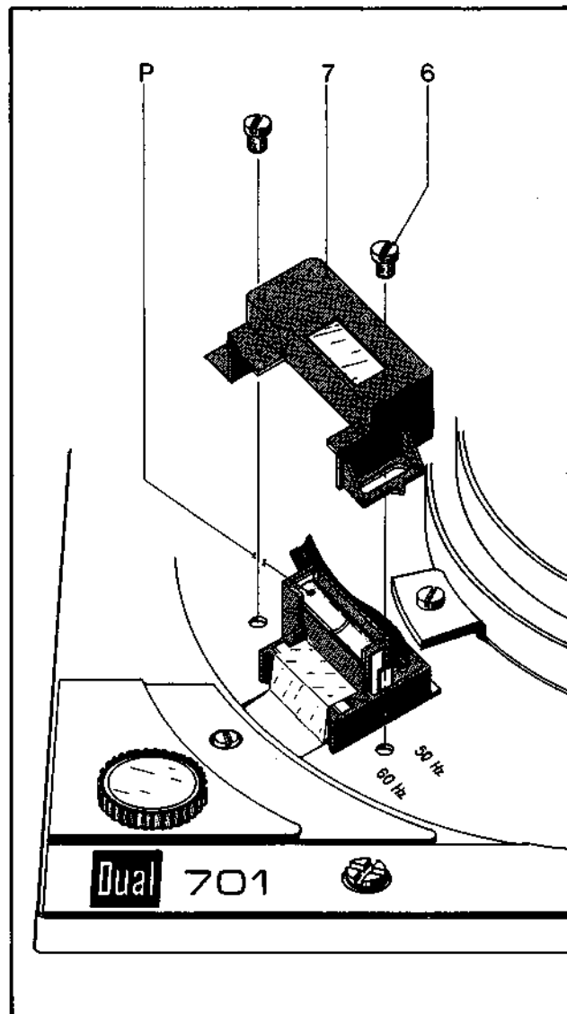
Fig. 9 Stroboskop
