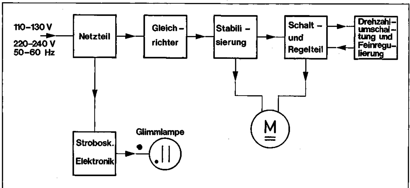
Fig. 4 Blockschaltbild
