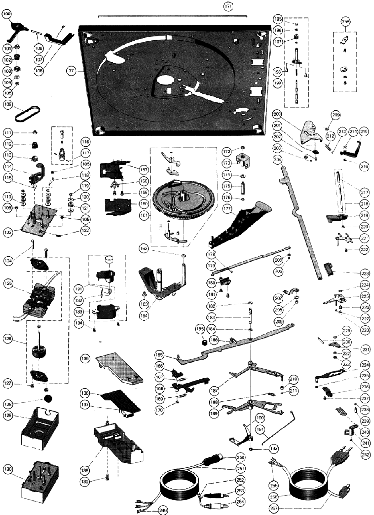
Fig. 20 Explosionsdarstellung 2
