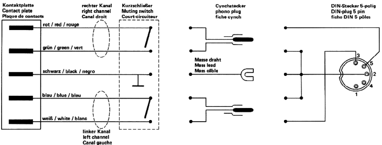
Fig. 1 TA-Anschlußschema
