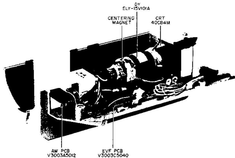
Fig. 4 EVF Block
