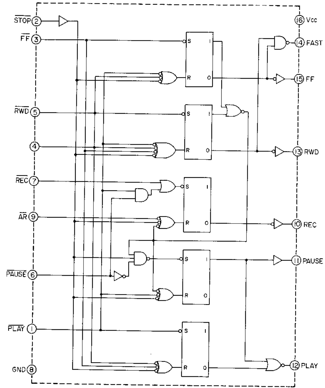
Fig. 4 M54410P
