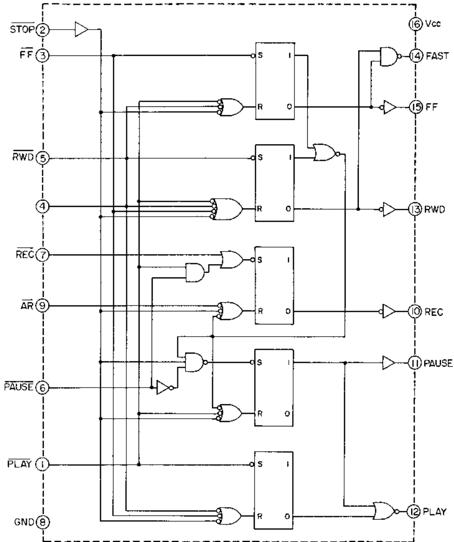
Fig. 5 M54410P
