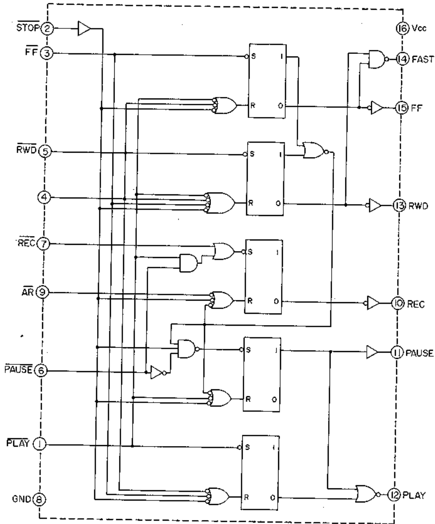
Fig. 6 M54410P
