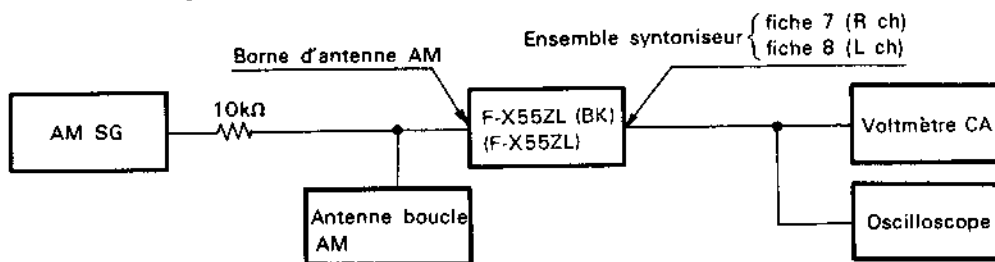
Fig. 12-2 Diagramme de raccordement de réglage MA
