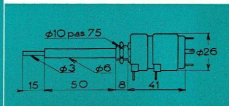
Double, axes indépendants avec inter.
