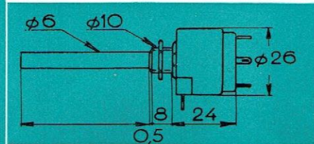
Simple avec interrupteur.
