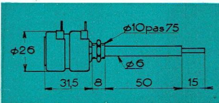
Double, axes indépendants sans inter.
