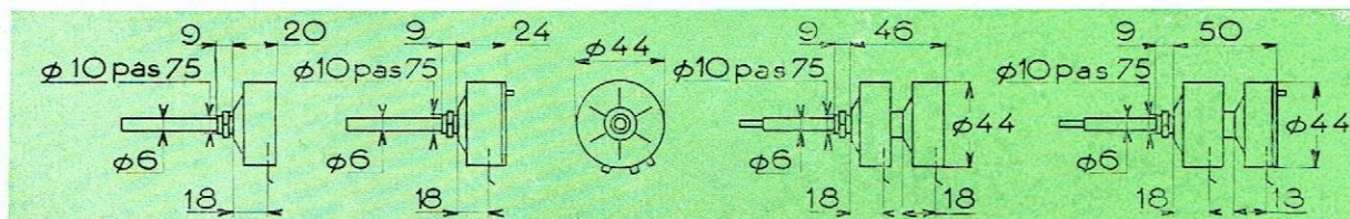
sans inter avec inter double sans inter double avec inter
