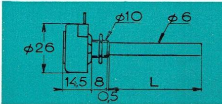
Simple sans interrupteur.
