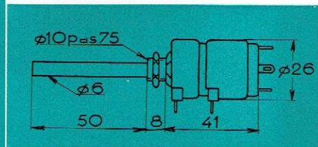
Double, axes jumelés avec inter.
