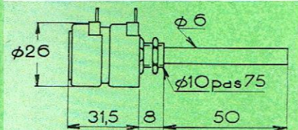
Double, axes jumelés sans inter.
