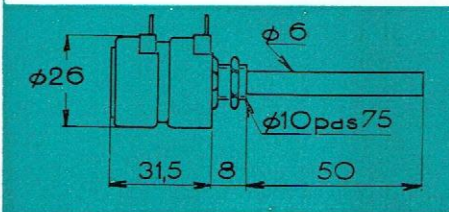
Double, axes jumelés sans inter.
