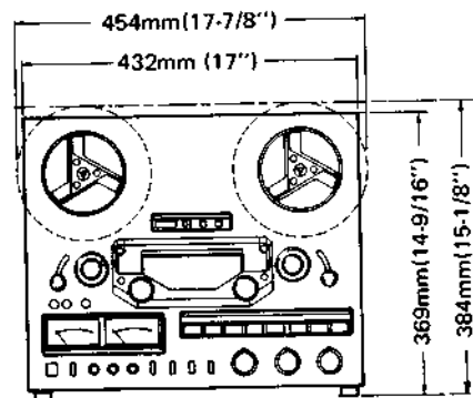
Fig. 1-1 Dimensions
