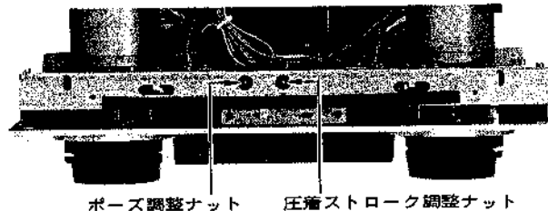
図2 ポーズ位置及び圧着ストローク調整個所
