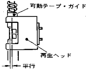
図14 再生ヘッドのあおり調整
