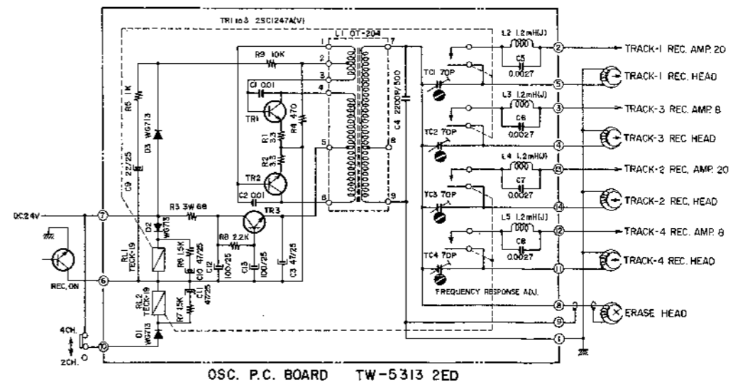
OSC. P.C. BOARD TW-5313 2ED
