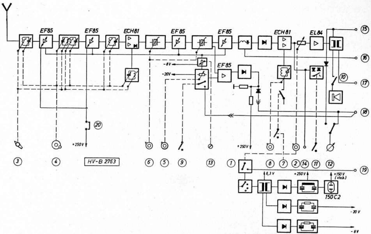
Abb. 2. Blockschaltbild des Kw-Empfängers E 127 Kw/4
