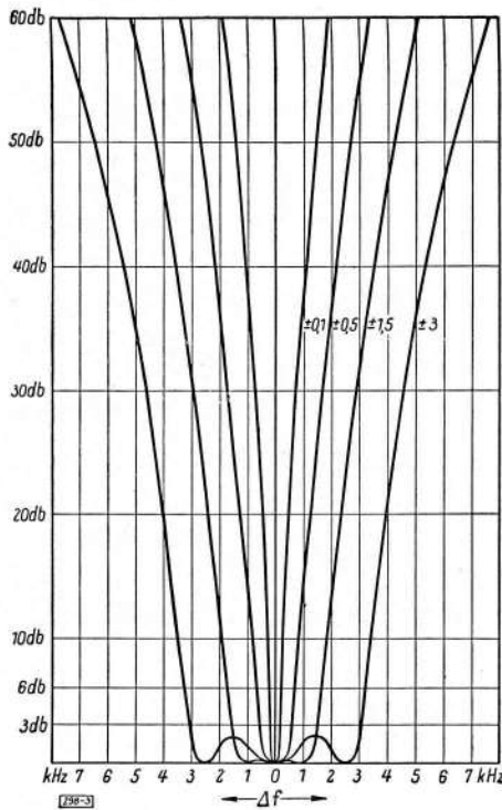
Abb. 9. ZF-Selektionskurven des Kw-Empfängers E 127 Kw/4 Als Parameter Bandbreite in kHz
