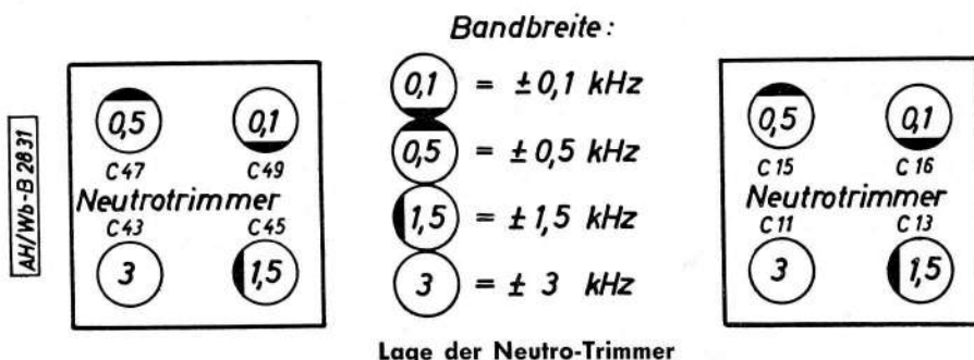
Abb. 8. ZF-Teil (2) Abgleichplan der 4 Bandbreiten
