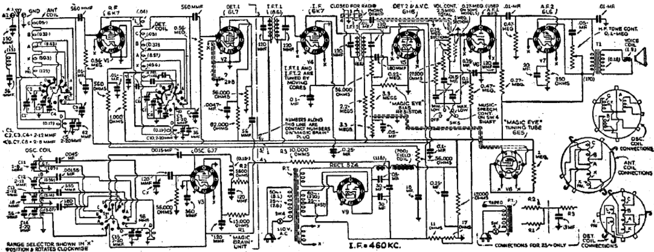
Supereterodina RCA modelli 9T e 9K2.
