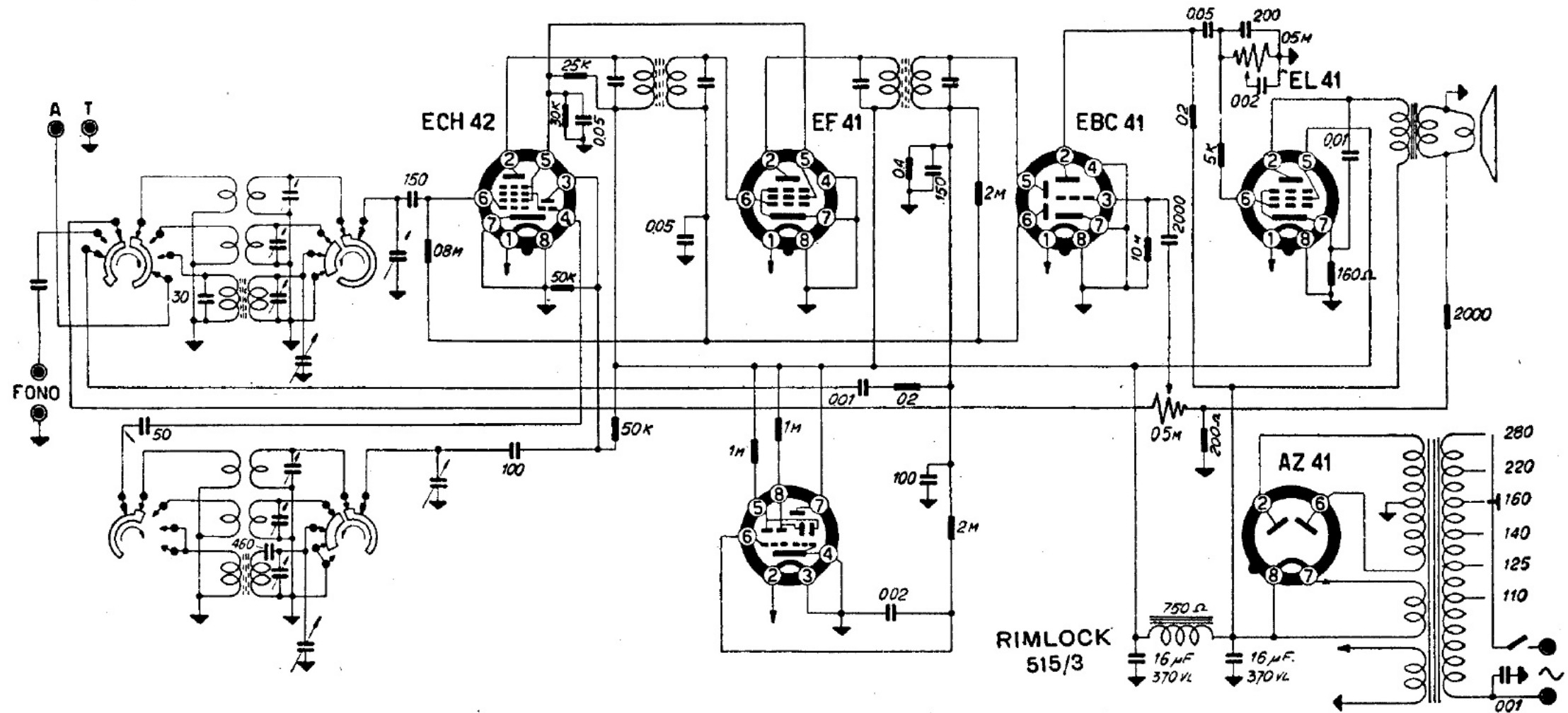
MINERVA RADIO - Mod. Rimlock 515/3. Onde medie e due corte. Media frequenza a 468 kc. Esiste un mod. 515/3 con valvole di tipo americano. Resa d'uscita 3 watt. Consumo 55 watt.
