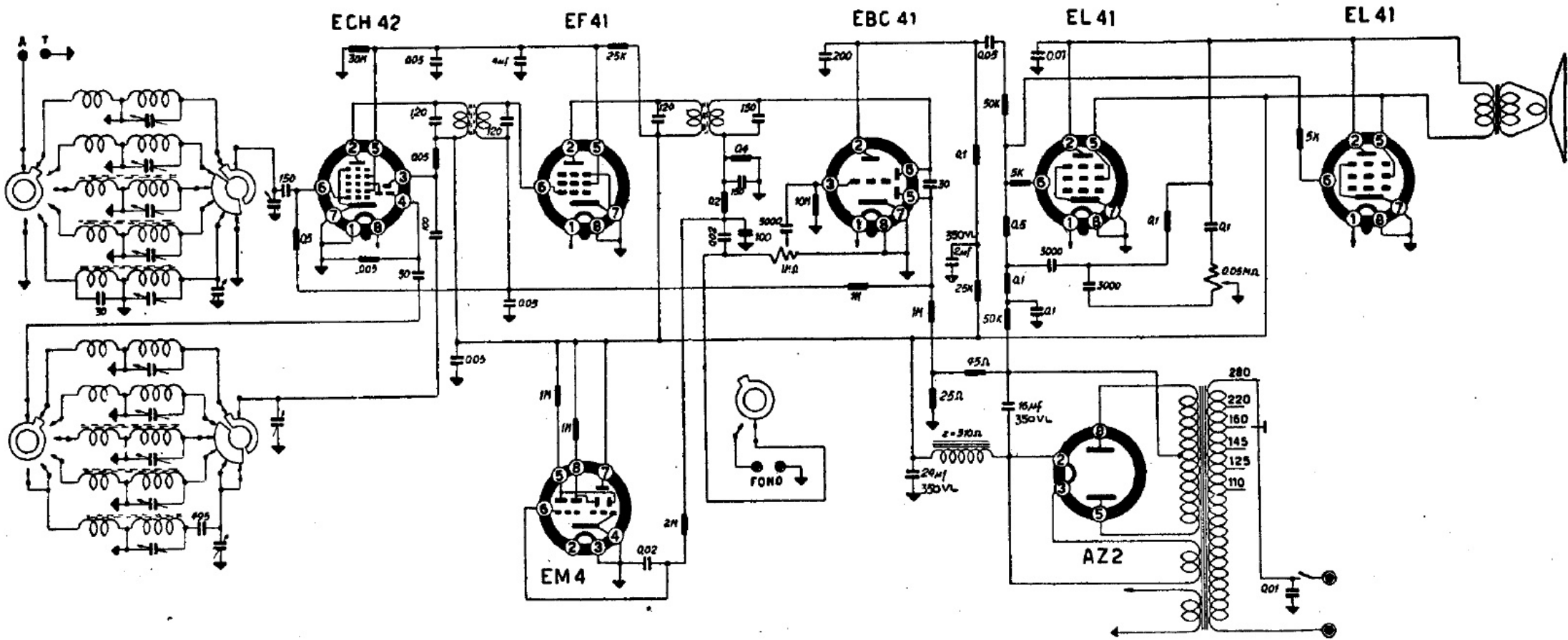
MINERVA RADIO - Mod. 506/1 - Medie e tre corte. Media frequenza 470 kc. Due EL41 in parallelo. Uscita 4,5 watt.
