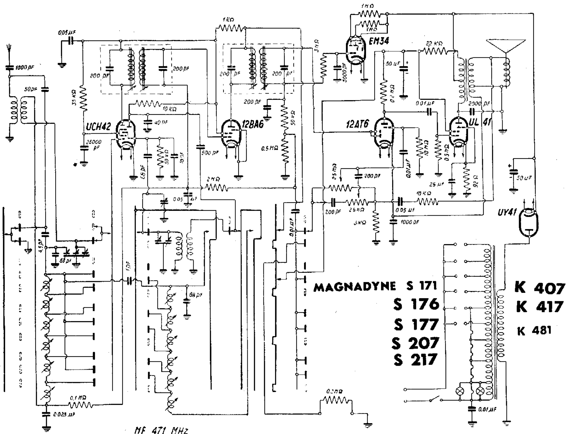
MAGNADYNE RADIO - Modd. MAGNADYNE S171, S176 ed S177; KENNEDY K481. Gamme onde medie e sei gamme allargate ad onde corte e cortissime. Media frequenza 471 kc/s. I modd. Magnadyne S207, S 217, Kennedy K407 e K417 differiscono dagli altri menzionati per avere le seguenti valvole: ECH81, 12P1, 12DT1, 35F4 e UY41.
