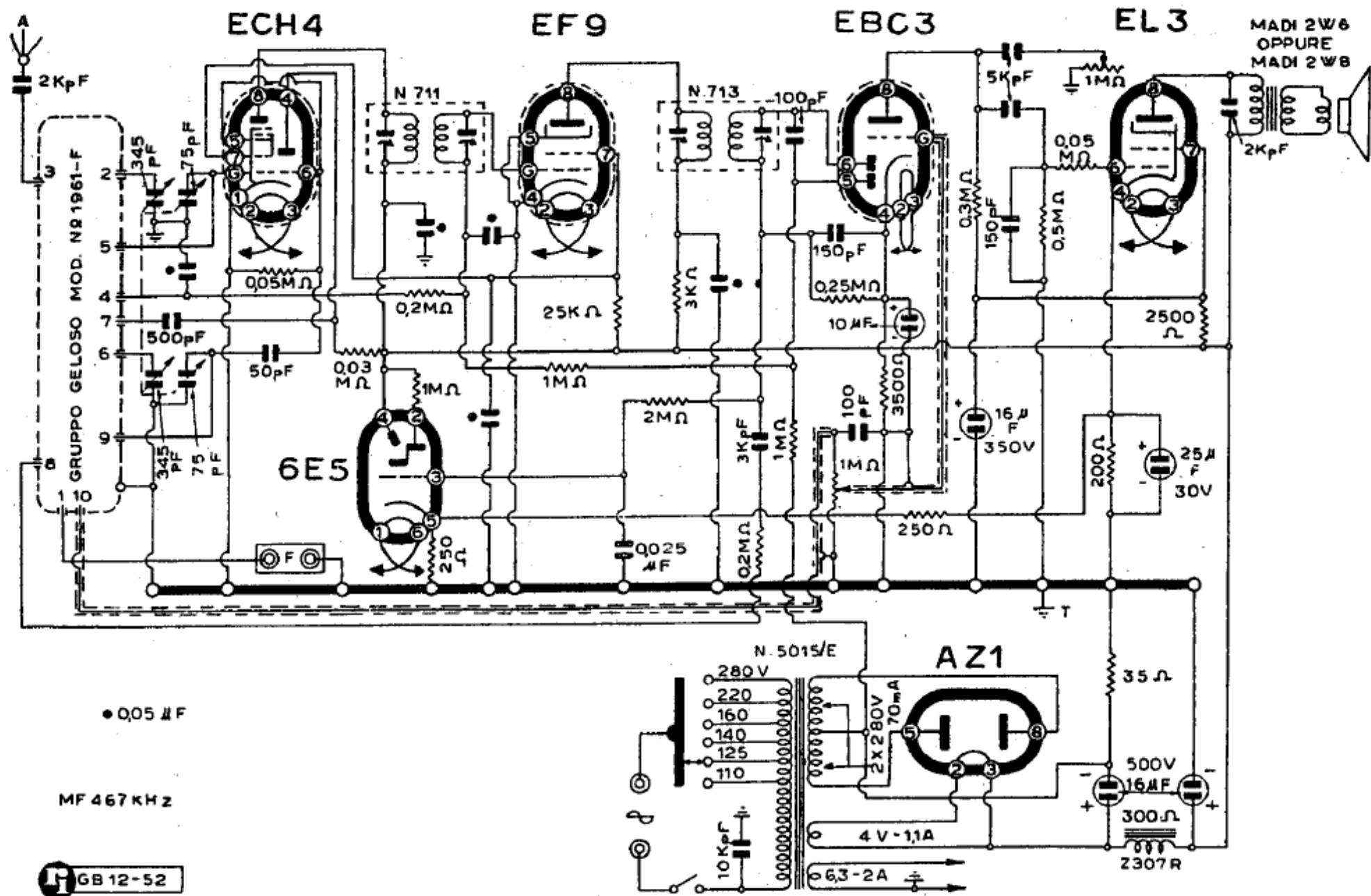
GELOSO S.A. - Modd. Super G 131/RE - G 504/RE
