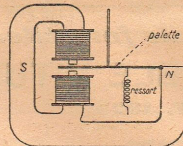
S.- Fig. 2 - Moteur à palette polarisée
