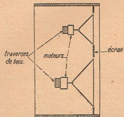
S... Fig. 10. Deux moteurs séparés.
