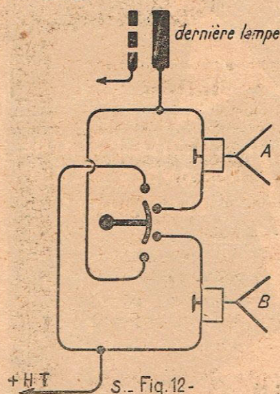
S... Fig. 12. Montage des 2 cônes
