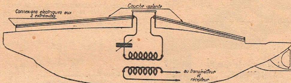
J.F.C. - Coupe du sous-marin avec le système ROGERS.
