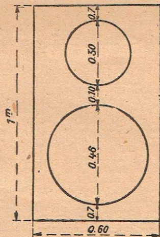
S... Fig. 11. Cotes de l'écran
