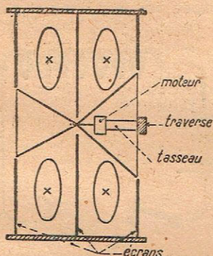
S... Fig. 7. Dispositif à un seul moteur
