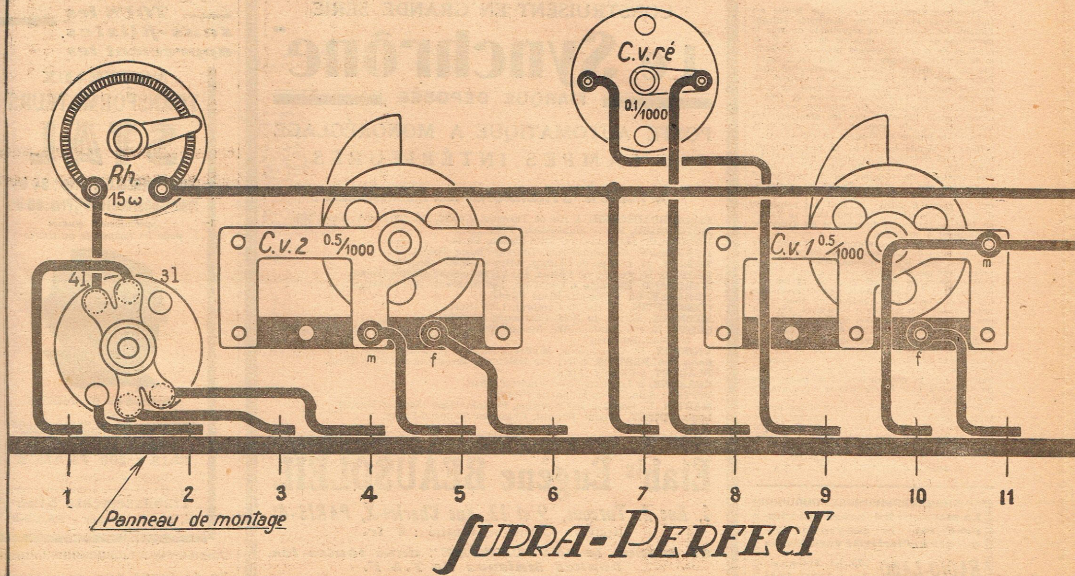
Panneau avant 420 x 210
