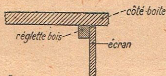
S... Fig. 8. Fixation d'un écran au boîtier.
