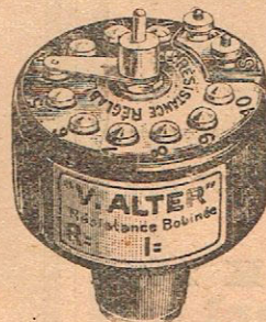
Résistance variable à plots B. 5.
